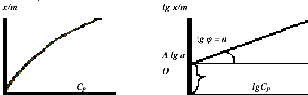
Рис.2. Изотерма адсорбции.
